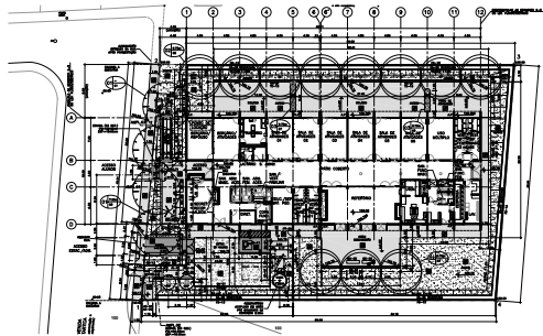
PLANTA DE IMPLANTAÇÃO
