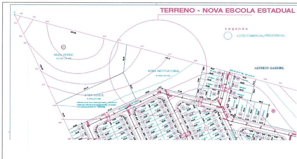
Planta localização do terreno onde será implantada a nova Escola Estadual
