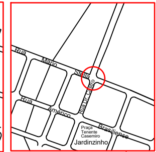
DETALHE 02 - CONJ. SEMAFÓRICO 03 FASES
