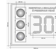
DETALHE 01 - CONJ. SEMAFÓRICO 04 FASES
