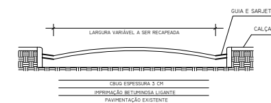
Corte transversal da rua
