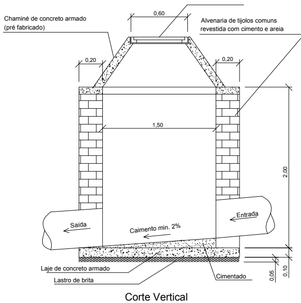
DETALHE DA CAIXA SEM ESC.
