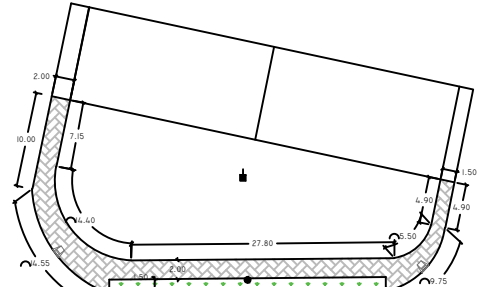
Planta calçada 05 Esc.: 1:500
