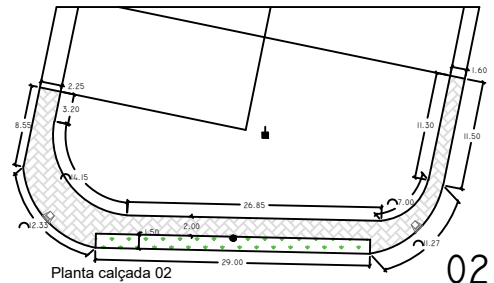
Planta calçada 02 Esc.: 1:500
