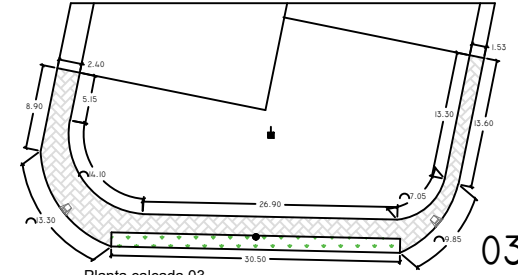
Planta calçada 03 Esc.: 1:500
