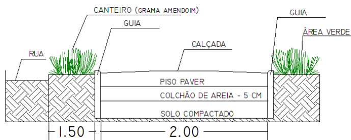
PERFIL EXPLICATIVO DAS CALÇADAS S/ESC.
